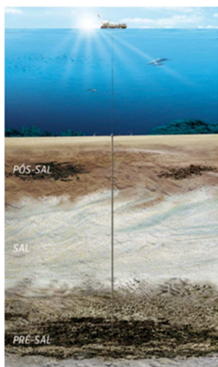
Figura 20 – Modelo das jazidas de pré-sal, formadas por depósitos de matéria orgânica acumulados por mais de 100 milhões de anos e que foram prensadas por camadas de sal depositadas no solo marinho (Fonte Petrobras: http://www.petrobras.com.br/pt/nossas-atividades/areas-de-atuacao/exploracao-e-producao-de-petroleo-e-gas/pre-sal/ ).
