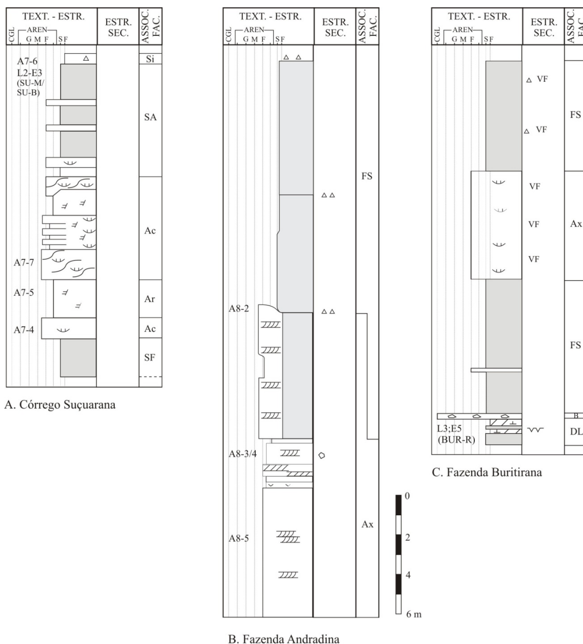
Figura 17. Perfis córrego Suçuarana, fazendas Andradina e Buritirana – Formação Motuca.
