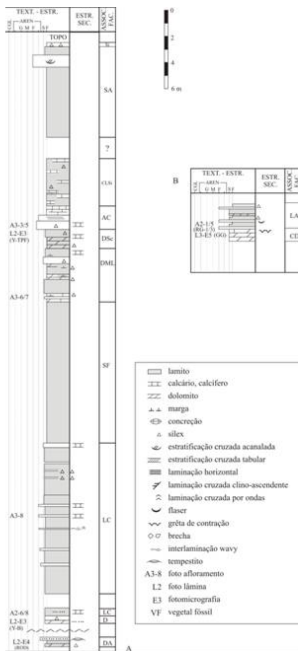
Figura 15. Perfis estratigráficos da porção oeste da área e oeste de Bielândia
