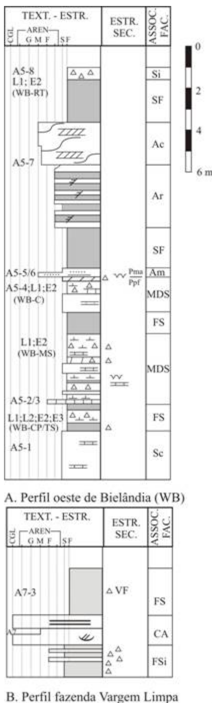
Figura 16. Perfis oeste de Bielândia e Vargem Limpa, formações Pedra de Fogo e Motuca.
