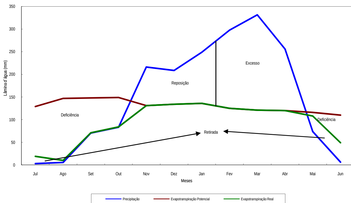
Figura 1. Curso anual normal do balanço hídrico do Monumento Natural das Árvores Fossilizadas do Estado do Tocantins, calculado pelo método de Thorntwaite & Mather, para 100 mm de capacidade de armazenamento.
