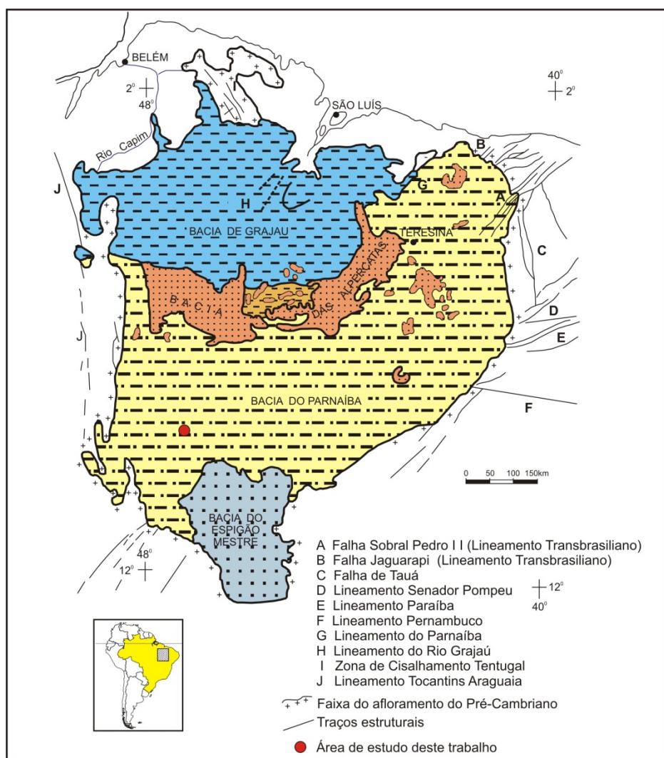
Figura 12. Compartimentação da Província Sedimentar do Meio-Norte do Brasil (GÓES, 1995; GÓES; COIMBRA,1996).
