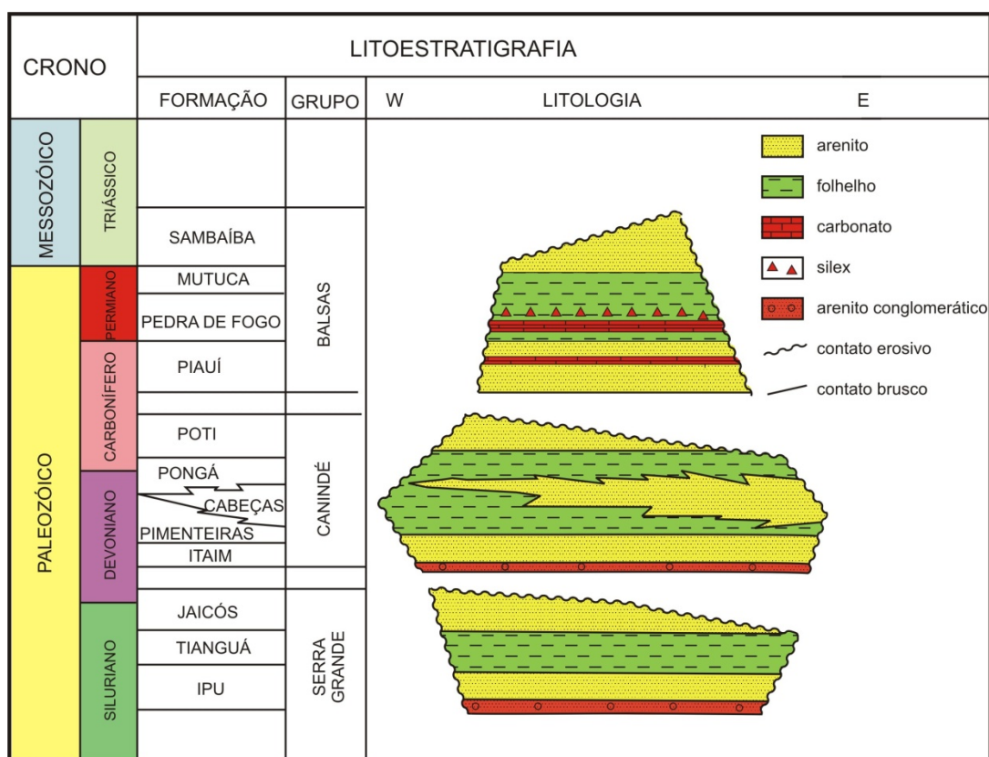
Figura 14. Coluna estratigráfica da Bacia do Parnaíba (GÓES, 1995; GÓES; COIMBRA, 1996).
