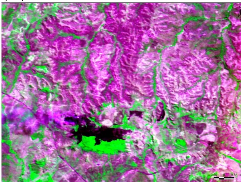
Figura 3. Resposta espectral dos terrenos do alto das sub-bacias do Ribeirão Arraias e Rio João Aires em imagens Cbers 2.
